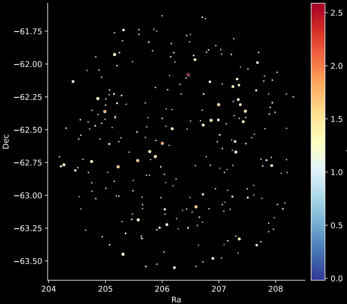
GALAH DR4 Field: [7165] Stars: 252
