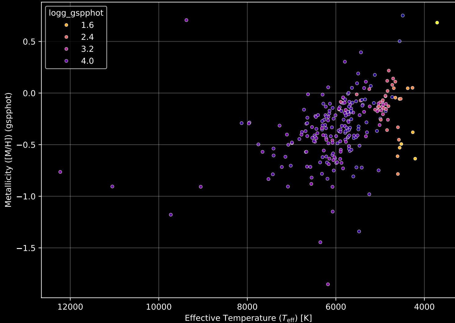
GALAH DR4 Field: [7165] Stellar Population Parameters (n= 252)
